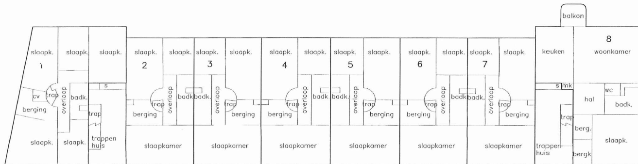
1e verdieping 1:100
