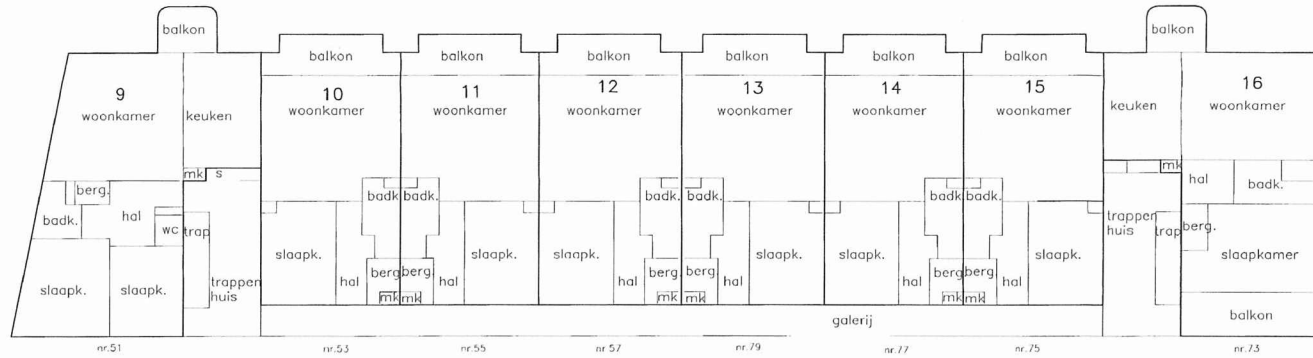
2e verdieping 1:100
